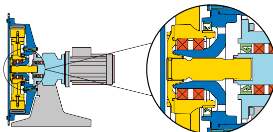
Acoplamiento directo Bredel
